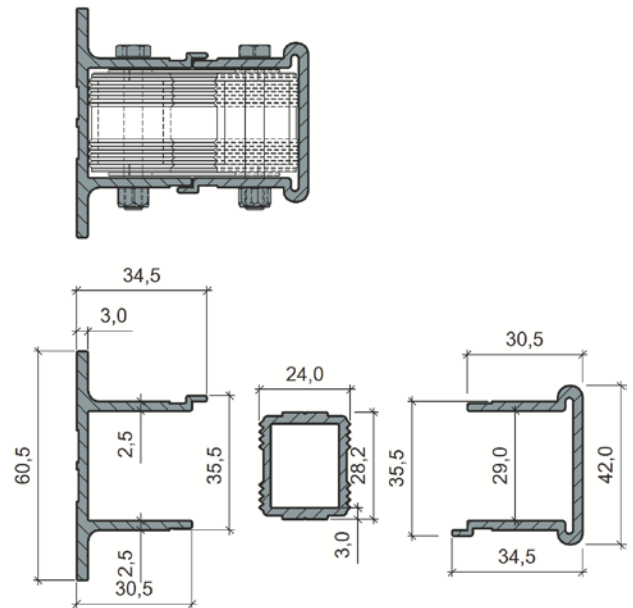
Fig. 5 Profiler til indre vange, trinn og ytre vange. Profilerne festes sammen med M5 x 40 mm trinnskruer og M5 låsemuttere.
