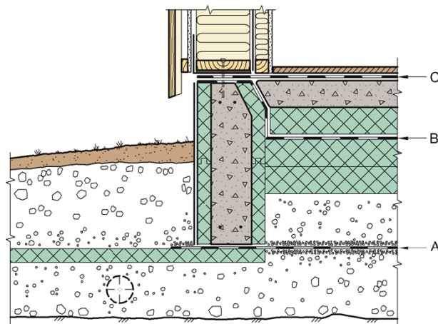
Fig. 1 Prinsipiell plassering av radonsperrer i ulike bruksgrupper. ULTIPRO Radonsperre er godkjent for bruksgruppe B og C.
