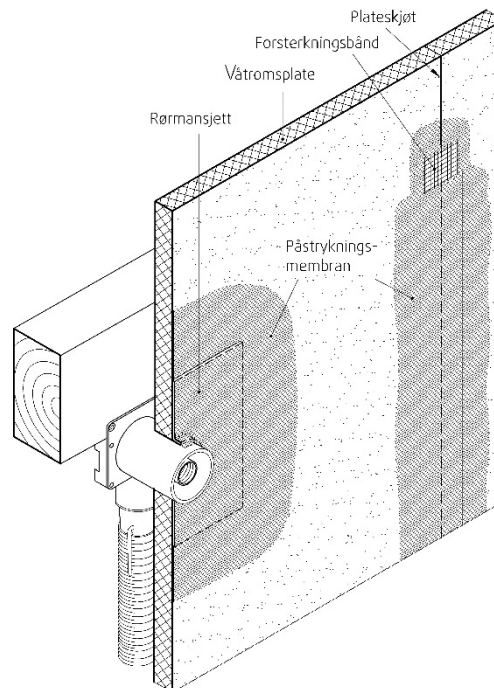
Fig. 1 Eksempel på våtromsplatesystem med tilhørende tettedetaljer
