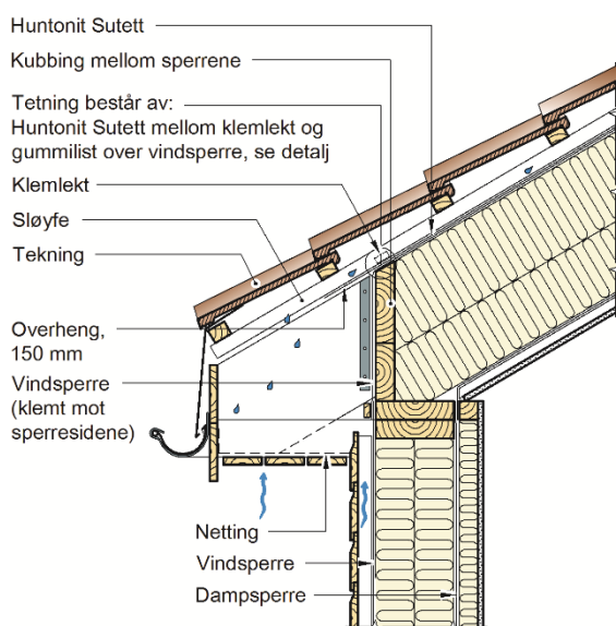
Fig. 4b Eksempel på utførelse med ikke kontinuerlig vindsperre. Ytterveggenes vindsperre fra veggene blir klemt mot Huntonit Sutett ved kubbingene mellom sperrer.
