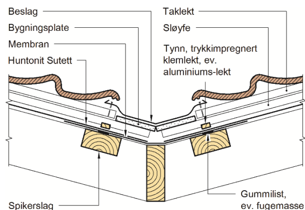
Fig. 6 Eksempel på detalj ved vinkelrenne. Overgangen mellom platene i de to takflatene skal gjøres lufttett ved å først legge en vindsperreduk.
