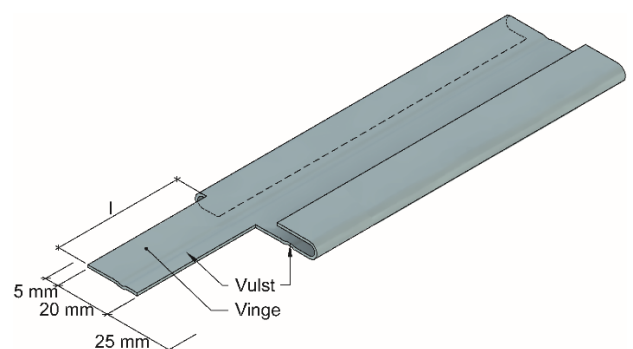
Fig. 2 Huntonit Sutettbeslag. Vingen leveres med lengde 36 eller 48 mm.
