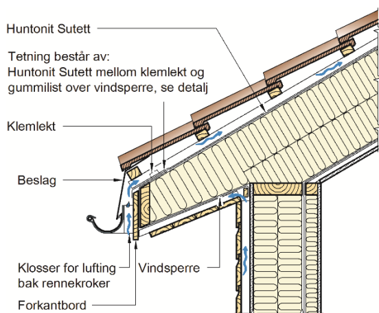
Fig. 4a Eksempel på utførelse med kontinuerlig vindsperre rundt raftekassen. Vindsperran blir ført rundt raftekassen.
