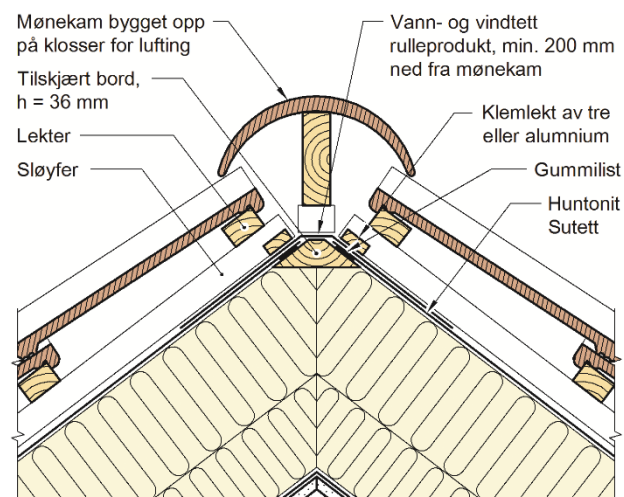
Fig. 7 Eksempel på mønedetalj. Overgangen mellom platene i de to takflatene skal gjøres lufttett ved å legge et rullbasert vindsperreprodukt som er klemt fast med klemlékte.
