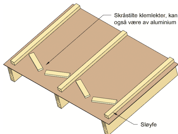
Fig. 5 Nedre klemlékt skal posisjoneres skrå for å unngå vannoppsamlinger. Klemlékt av stål eller aluminium er også en adekvat løsning og beskrevet i Byggforskserien.
