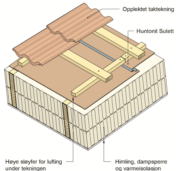
Fig. 1 Prinsipiell oppbygning av skrå tretak med Huntonit Sutett kombinert undertak og vindsperre alltid i forbindelse med Huntonit Sutettbeslag.
