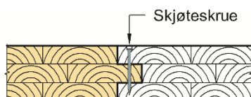
Fig. 4 Prinsipp for elementskjøt mellom overlappende elementer. Normal skruavstand er 600 - 800 mm.
