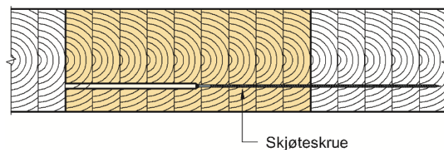
Fig. 5 Prinsipp for elementskjøt mellom kantstilte elementer. Normal skruavstand er 800 mm.
