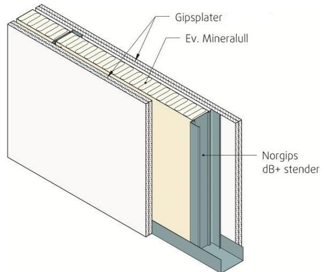
Fig. 1 Prinsipiell oppbygning av Norgips Skilleveggsystem.
