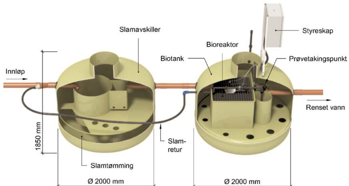
Fig. 1 Oversiktsskisse av renseanlegget (1 hh)
