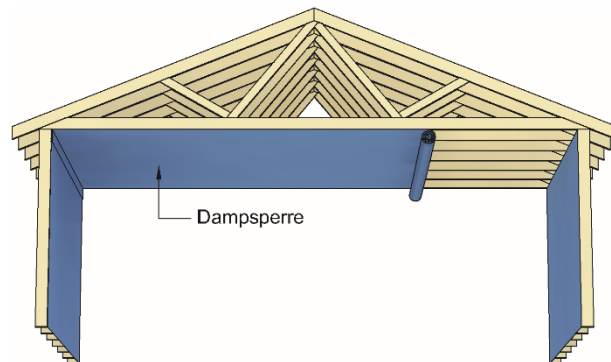
Fig. 1 Kullaplast Dampsperre montert i yttervegger og mot kaldt loftstom
