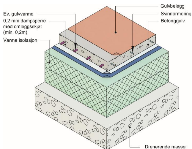
Fig. 3 Kullaplast Dampsperre montert i betonggolv på grunnen
