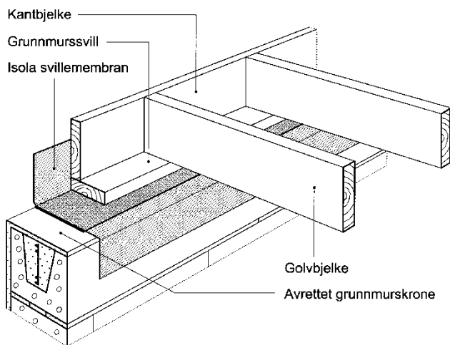
Fig. 2 Eksempel på bruk av Isola Svillemembran med asfaltbredde 20 cm montert på grunnmur til kjeller eller kryperom.
