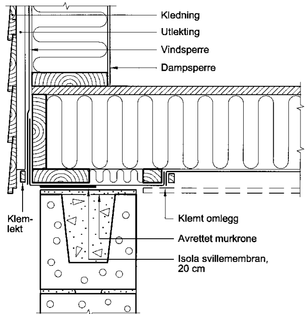
Fig. 3 Eksempel på bruk av Isola Svillemembran ved etasjeskiller på grunnmur. Ved bruk av murblokker skal murkronen være pusset før membranen blir lagt. Hvis det brukes bredere sviller enn 148 mm kan 20 cm, 25 cm eller 30 cm svillemembran benyttes og vindspærrefliken brettes tilbake under svillen.
