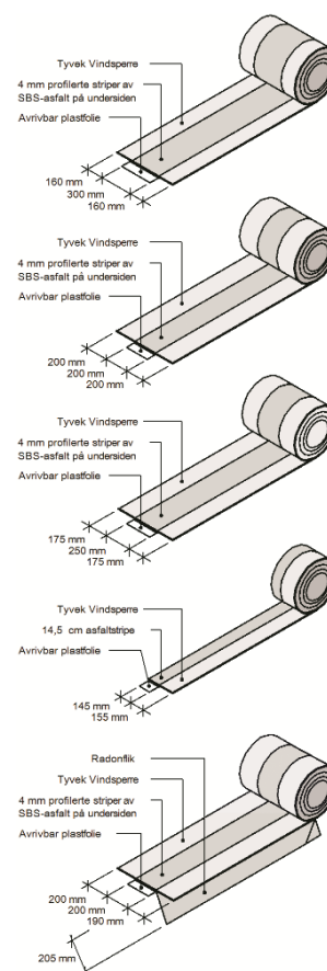
Fig. 1 Isola Svillemembran. Membranen leveres i fire forskjellige bredder tilpasset ulike veggtykkelser og tilslutninger ved fundament som vist i eksemplene i fig. 2, 3 og 4.
