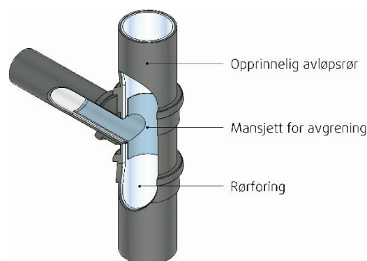
Fig. 1 Oppbygning av Boldan In-House Lining System
