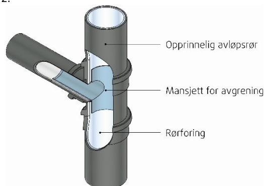
Fig. 1 Oppbygning av Houseliner System
