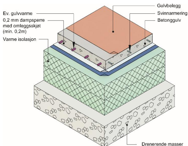
Fig. 3 Protan Dampsperre monteret i betonggolv på grunnen
