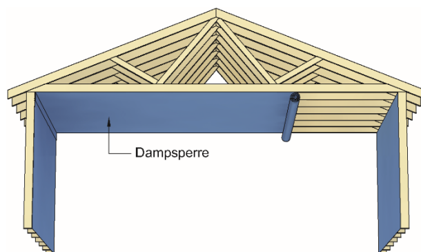
Fig. 1 Protan Dampsperre monteret i yttervegger og mot kaldt loftsrom
