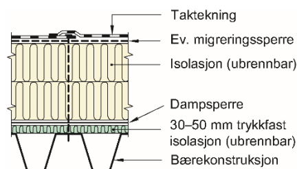
Fig. 2 Protan Dampsperre monteret i kompakt takkonstruksjon
