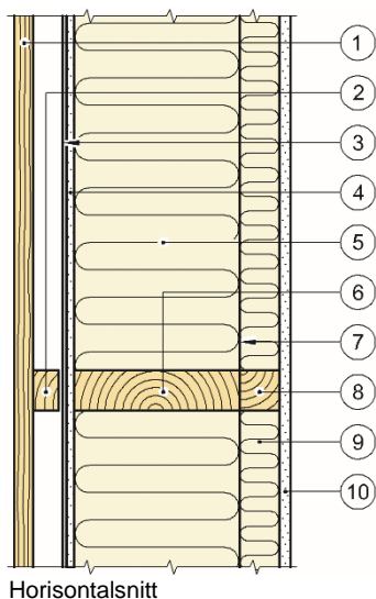
Horisontalsnitt
