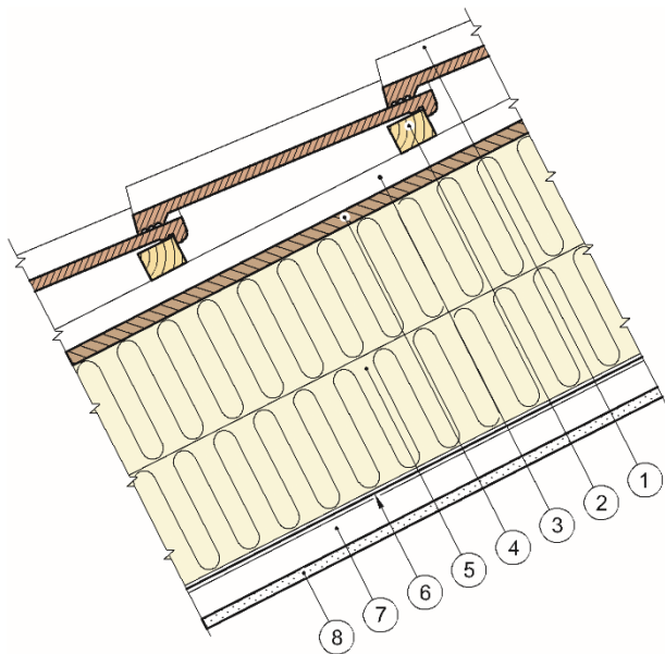
Vertikalsnitt
