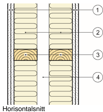
Horisontalsnitt
